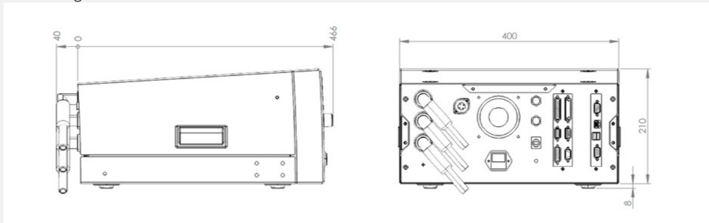
Abmessungen Gehäuse mit Winkelsteckern:
