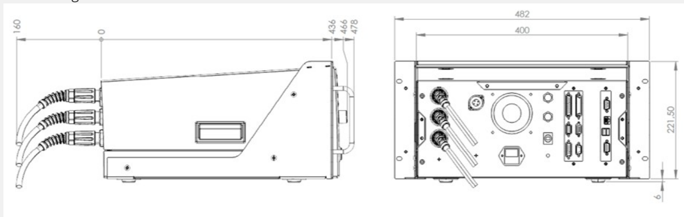
Abmessungen Gehäuse mit Einbausatz 19 Zoll:
