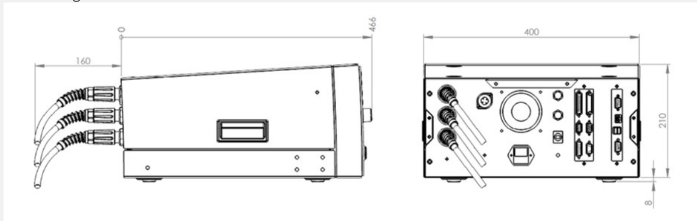
Abmessungen Gehäuse:
